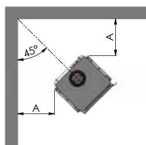
1446/1448 hoekinstallatie
