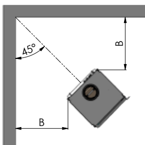
1416/1418 hoekinstallatie
